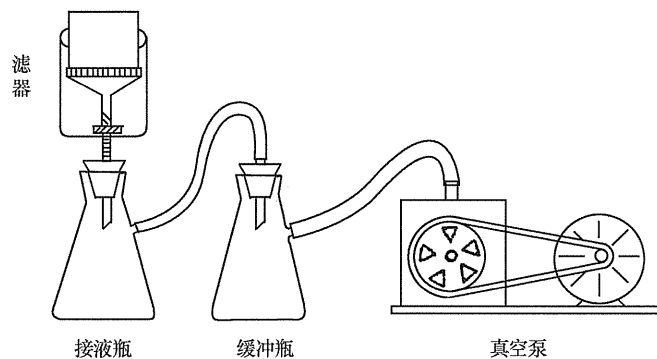
图 1 过滤装置
