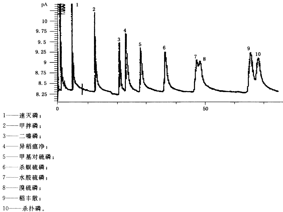
图 2 10 种有机磷气相色谱图
