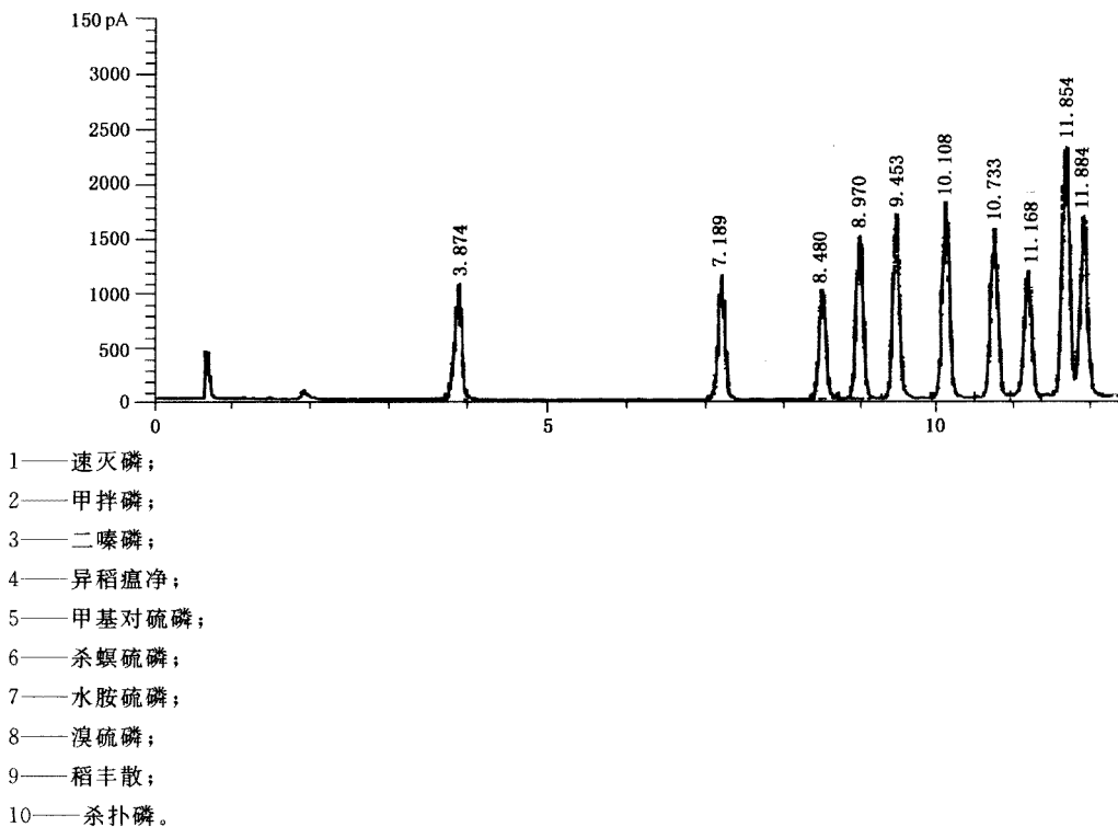
图 3 10 种有机磷气相色谱图
