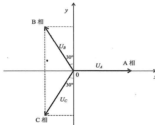
图 C.1 对地电压计算图
