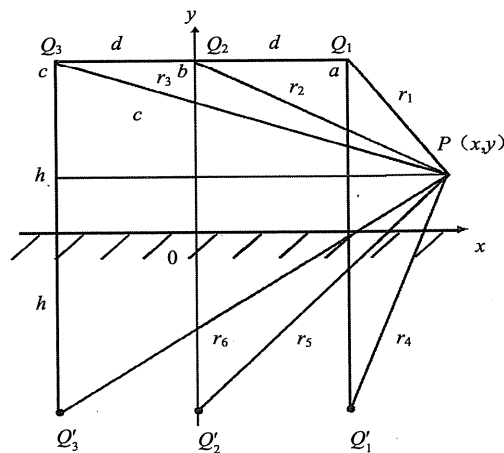
图 C.5 各导线坐标图
