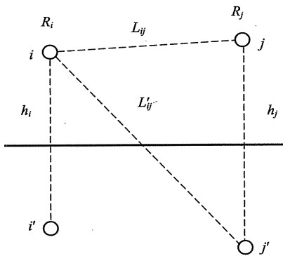
图 C.2 电位系数计算图
