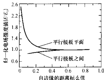
图 A.1 处于平行极板表面和平行极板中间的归一化的电场值（标么值表示）
